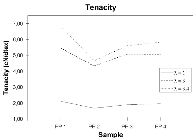
Figure 2: Tenacity of samples Slika 2: Pretržna napetost vzorcev
