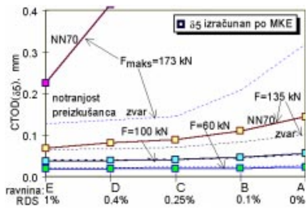
Slika 8: Primerjava med izračunanimi vrednostmi CTOD( \delta_5 ) za nionicral 70 in visokotrnostni strjeni zvar
