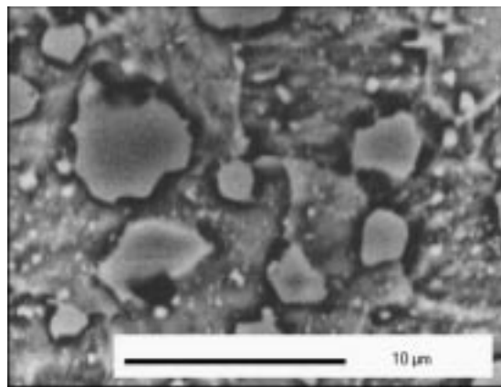
Slika 7: M 7 C 3 faze, Z-contrast in EDS spekter
