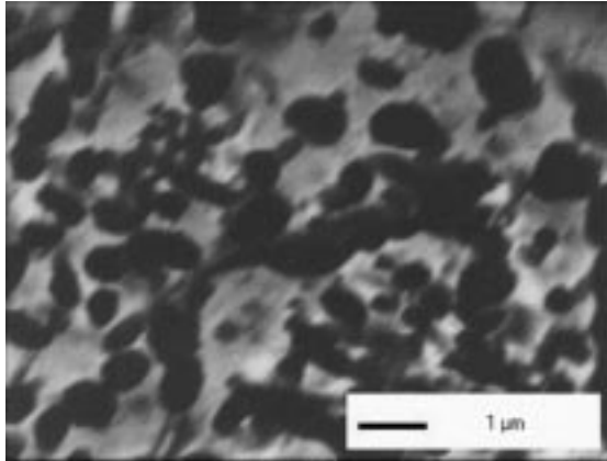
Slika 6: Fe 3 C faze, Z-contrast in EDS-spekter
