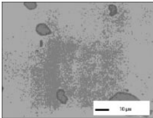
Slika 5: MnS vključki, Z-contrast in EDS-spekter
