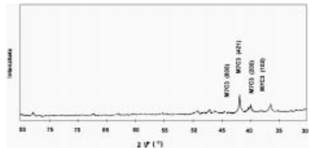
Slika 8: Rentgenogram karbidne faze M 7 C 3 v jeklu OCR12
