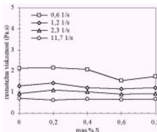
Slika 4: Odvisnost ravnotežne viskoznosti od koncentracije surfinola E104 (vzorec ni vseboval bentona 38) pri štirih različnih strižnih hitrostih Figure 4: Dependence of equilibrium values of viscosity on concentration of Surfinol E104 (for sample without Bentone 38) at four different shear rates
