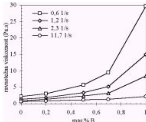
Slika 3: Odvisnost ravnotežne viskoznosti od koncentracije bentona 38 (vzorec ni vseboval surfinola E104) pri štirih različnih strižnih hitrostih Figure 3: Dependence of equilibrium viscosity on concentration of Bentone 38 (for sample without Surfinol E104)
