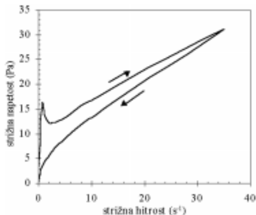
Slika 1: Tokovna krivulja kot rezultat trikotne metode za vzorec, ki je vseboval 0,8 mas.% surfinola E104 in 0,7 mas.% bentona 38 Figure 1: Flow curve as a result of triangular metod for sample with 0.8 wt.% of Surfinol E104 and 0.7 wt.% of Bentone 38
