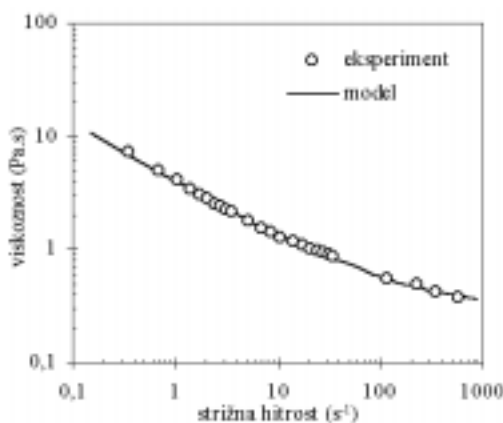
Slika 2: Viskozni profil za vzorec, ki je vseboval 0,8 mas.% surfinola E104 in 0,7 mas.% bentona 38: primerjava eksperimentalnih podatkov (točke) z izračunanimi vrednostmi (krivulja) na podlagi reološkega modela Sisko Figure 2: Viscosity curve for sample with 0.8 wt.% of Surfinol E104 and 0.7 wt.% of Bentone 38: the comparison between experimental points and calculated curve according to rheological model by Sisko
